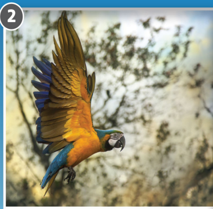
fly
